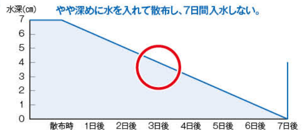
水管理のイメージ図(減水深1cm/日の場合)
